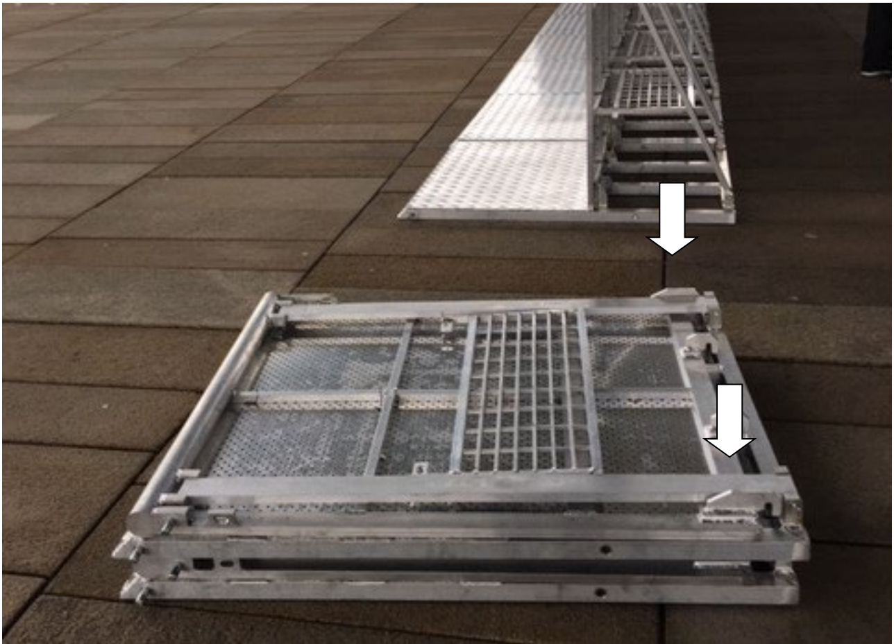
De staplas helt platt, och "låser" i varandra när de staplas (vit pil), så de är lätta att arbeta med och transportera på en Europall. De glider inte ner som andra system.
