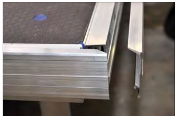
Verblendungsleisten einhängen
