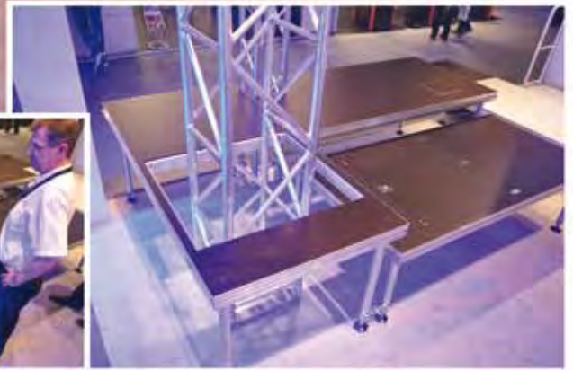
Podest mit Öffnung und Deckel
